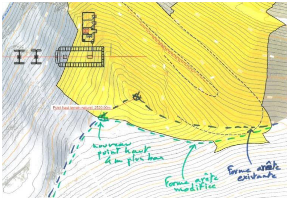
Schéma permettant de visualiser l'évolution de l'arête au niveau de la pointe des Chaudannes
